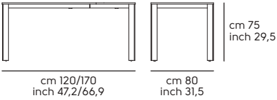
Blade 120/170x80
