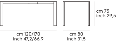
Badù 120/170x80
