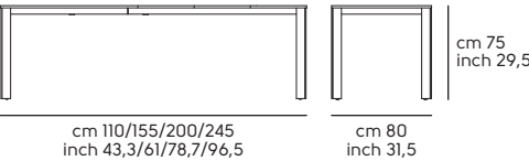
Blade 110/155/200/245x80
