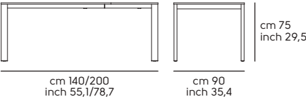
Badù 140/200x90
