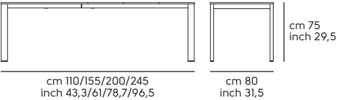
Badù 110/155/200/245x80
