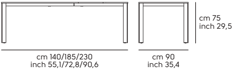
Blade 140/185/230x90
